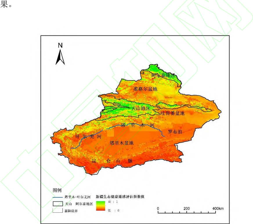
图 3 2018 年新疆生态健康遥感评估指数示意图 Fig.3 Ecological quality evaluation index of Xinjiang in 2018
