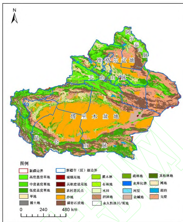
图1 新疆土地覆盖分类示意图
