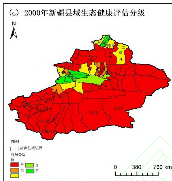
图 4. 各年县域生态健康遥感评估分级示意图
