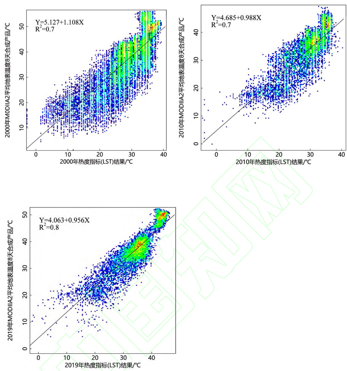
图 7 反演的 2000 年、2010 年和 2019 年的 LST 数据与 MOD11A2 产品的比较 Fig.7 Comparison of LST results with MODIS surface temperature products in 2000、2010 and 2019
