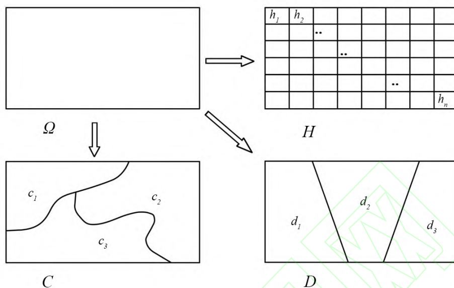
图 2 地理探测机理示意图
