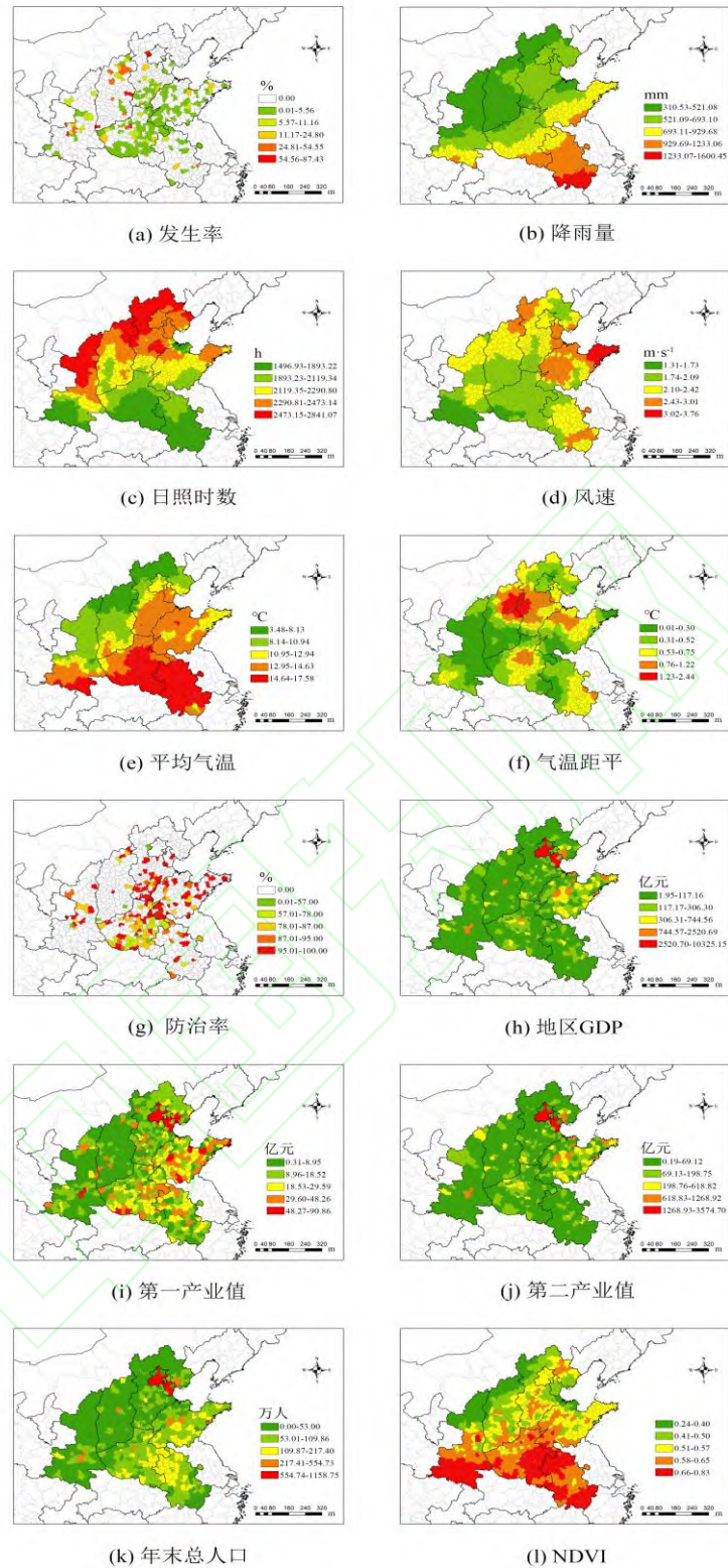
图3 华北地区（北京、天津、河北、山东、山西、陕西、安徽、河南八省市）光肩星天牛发病率与各自然社会经济指标空间分布图
