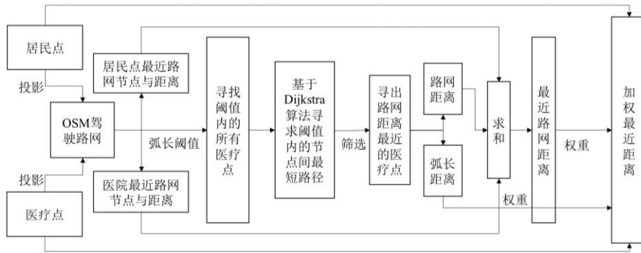
图2 OSMNHDC方法处理流程
