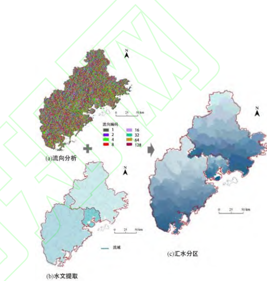
图 3 汇水区划分
