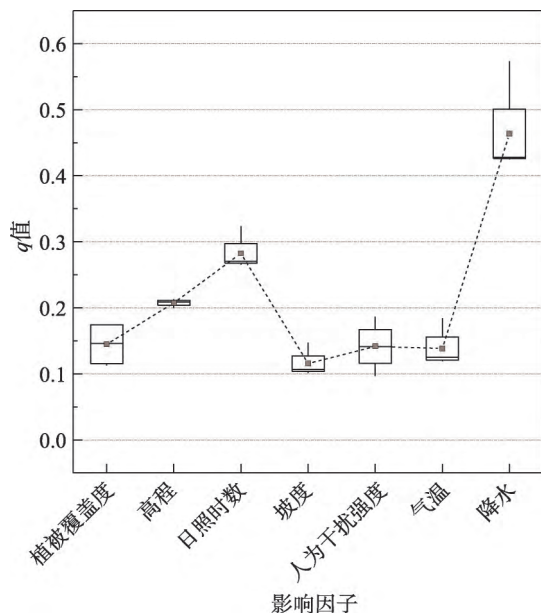
图3 疏勒河流域2001—2015年各驱动力因子解释度( q 值)箱线图
