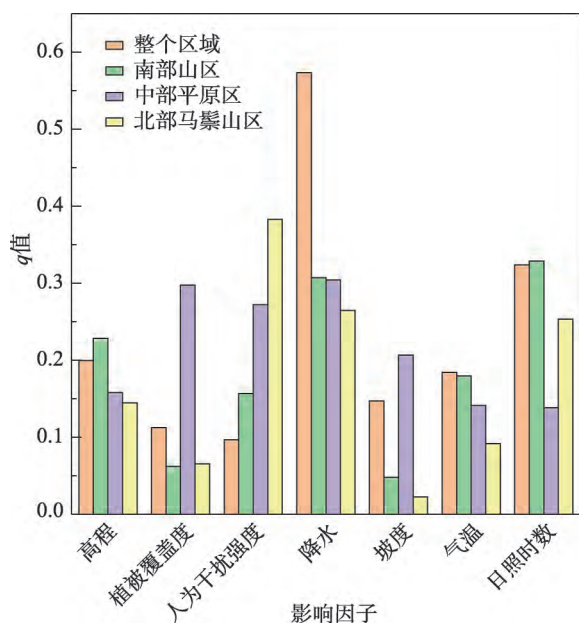
图4 疏勒河流域不同地理分区因子解释度( q 值)
