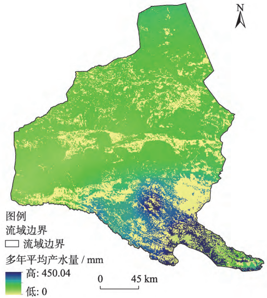
图2 疏勒河流域2001—2015年平均产水量空间分布 Fig. 2 Spatial pattern of annual average water yield in the Shule River Basin during 2001—2015
