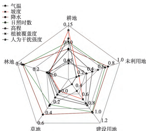
图6 疏勒河流域不同土地利用类型的因子解释度
