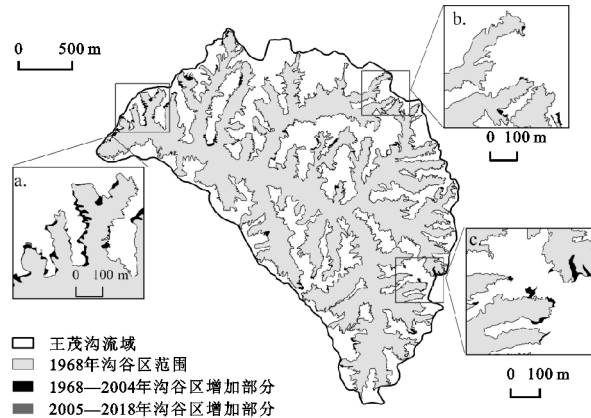
图 7 2 个时期沟谷区变化状况
