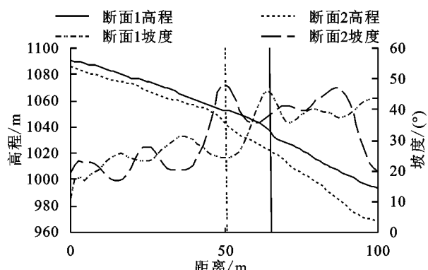
图4 断面剖面
