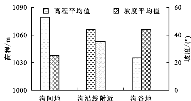
图5 正负地形高程和坡度统计
